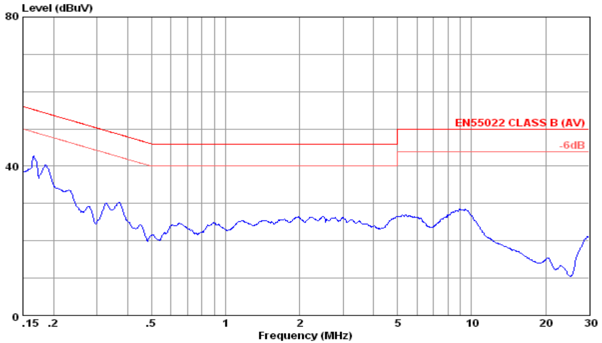
AV curve
